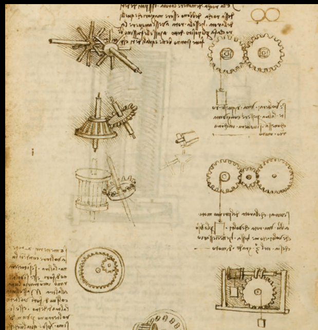
Foli f 15v. Codex Madrid I (Mss. 8937) "Tratado de estática y mecánica", 192 folios (384 pág.); format interior: 215 x 145 mm. Mecànica aplicada (màquines i enginyers). Mecànica aplicada (components). Principis de mecànica, cinemàtica, dinàmica. Crèdit: Album
